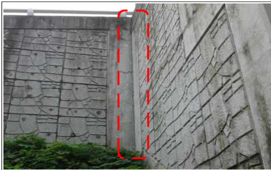
교대 A1 날개벽 실란트 손상
